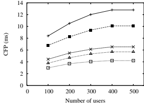
Fig. 7. Multicast AP=50.
